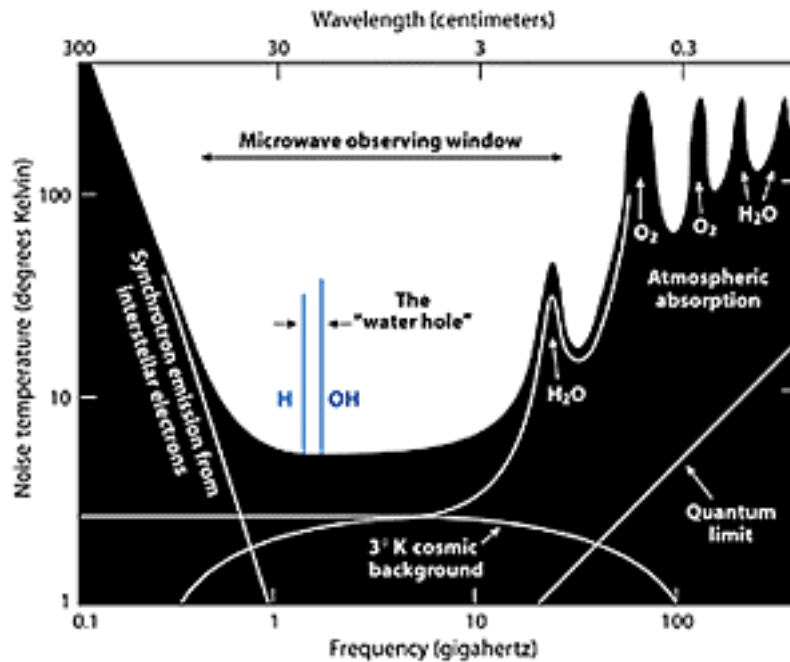
Fig. 3: Finestra radio utilizzabile per le ricerche SETI.
