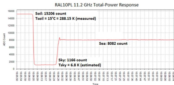
Fig. 20: Tipica escursione dinamica di un radiometro che misura il terreno, il cielo allo zenit e la superficie del mare.
