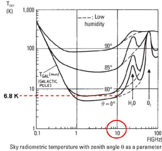
Fig. 19: Stima della temperatura di brillantezza del cielo allo zenit nella banda 12 ÷ 12 GHz (N. Skou, D. Le Vine - MICROWAVE RADIOMETER SYSTEMS - Design and Analysis).
