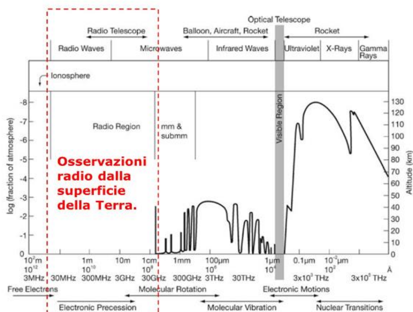
Fig. 4: Rappresentazione dello spettro elettromagnetico dove è stata evidenziata la “finestra radio”.
