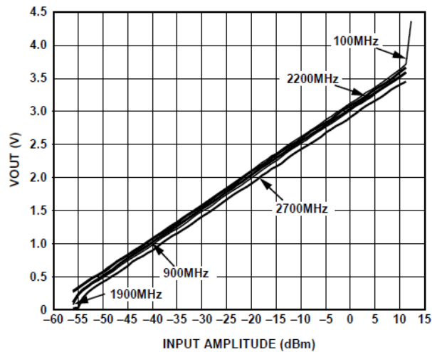
Fig. 13: Caratteristica ingresso-uscita del rivelatore compensato in temperatura AD8362 utilizzato nel radiometro RAL10MW .
