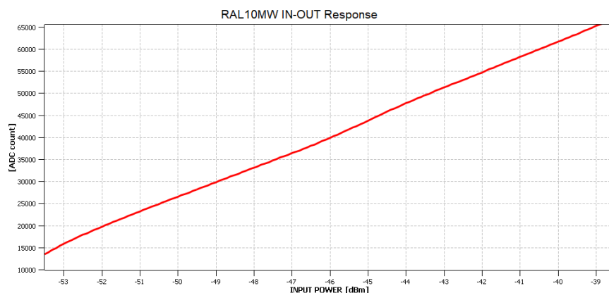
Fig. 16: Caratteristica ingresso-uscita del radiometro RAL10MW ottenuta in laboratorio applicando all’ingresso dello strumento un segnale sinusoidale a 1415\text{ MHz} e variando la sua potenza da -55\text{ dBm} fino a -38\text{ dBm} . Il radiometro è stato impostato con il minimo guadagno di post-rivelazione ( GAIN = 0 ) e una costante di integrazione TCOST = 8 . E’ stato annullato l’offset per la linea di base ( ZERO\_BASE = 0 ) e le misure sono iniziate dopo che lo strumento si è termicamente stabilizzato alla temperatura di regime ( TREF = 50\text{ }^\circ\text{C} ).
