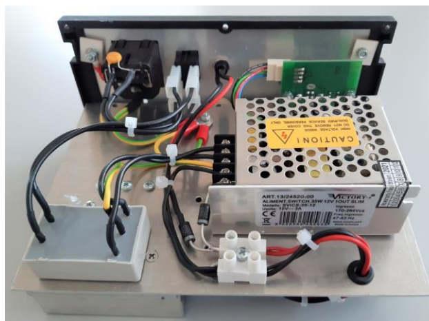
Fig. 15: Sezione di alimentazione da rete ( 230\text{ Vac} - 50/60\text{ Hz} ) del radiometro. E' disponibile un ingresso a bassa tensione ( 12\text{ Vdc} ) che consente di alimentare lo strumento tramite batterie esterne per utilizzi "sul campo".
