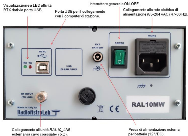
Fig. 1: Pannello frontale e posteriore del radiometro RAL10MW .
