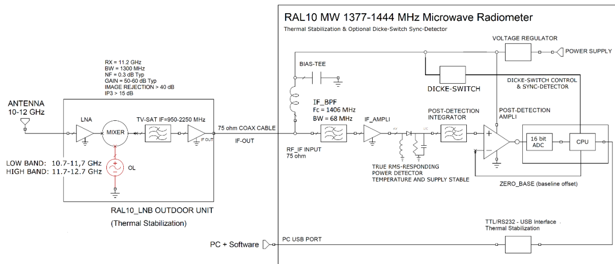
Fig. 12: Schema a blocchi che descrive i principali componenti di un radiotelescopio didattico operante nella banda 10 \div 12 GHz basato sul radiometro RAL10MW . Il blocco a sinistra rappresenta l'unità esterna (LNB) commerciale, completa di illuminatore, assemblata sul punto focale di un'antenna a riflettore parabolico (primo fuoco od offset) comunemente utilizzata per la ricezione TV-SAT. Il segnale a frequenza intermedia 950 \div 2250 MHz proveniente dall'unità esterna è trasmesso al radiometro RAL10MW attraverso un cavo coassiale da 75 \Omega , amplificato ed elaborato dal ricevitore, trasmesso al computer di stazione attraverso una porta seriale USB.
