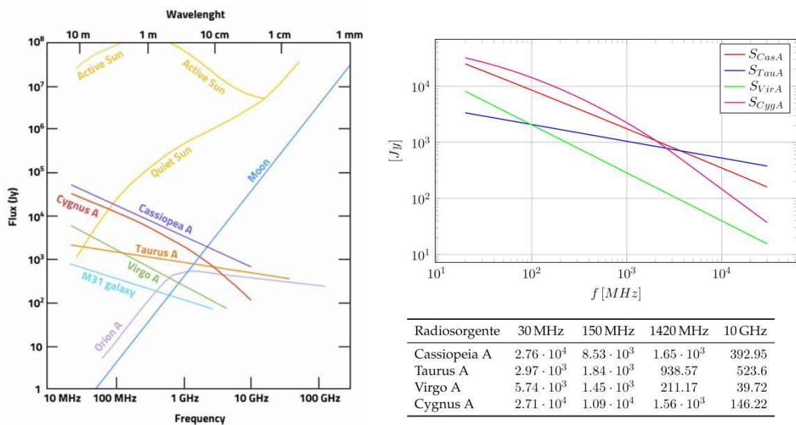
Fig. 7: Spettri delle principali radiosorgenti.
