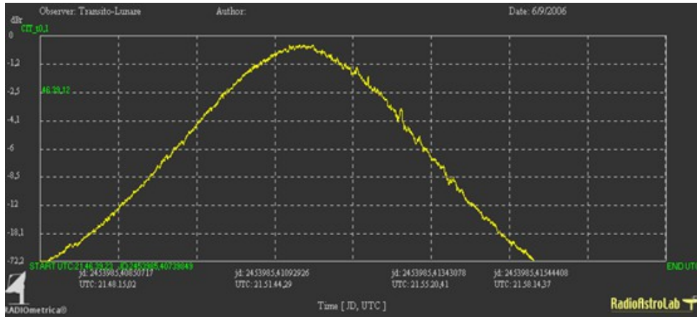
Fig. 19: Graphique d'un transit lunaire. Le rayonnement thermique de la lune est visible: son émission est le résultat du fait que l'objet émet approximativement comme un corps noir, caractérisé par une température de l'ordre de 300 K. Si l'émission visible de la Lune est presque exclusivement en raison de la lumière réfléchie du Soleil, dans le 11.2 GHz il y a un problème en raison de la température de l'objet qui contraste avec celle du ciel "à froid".
