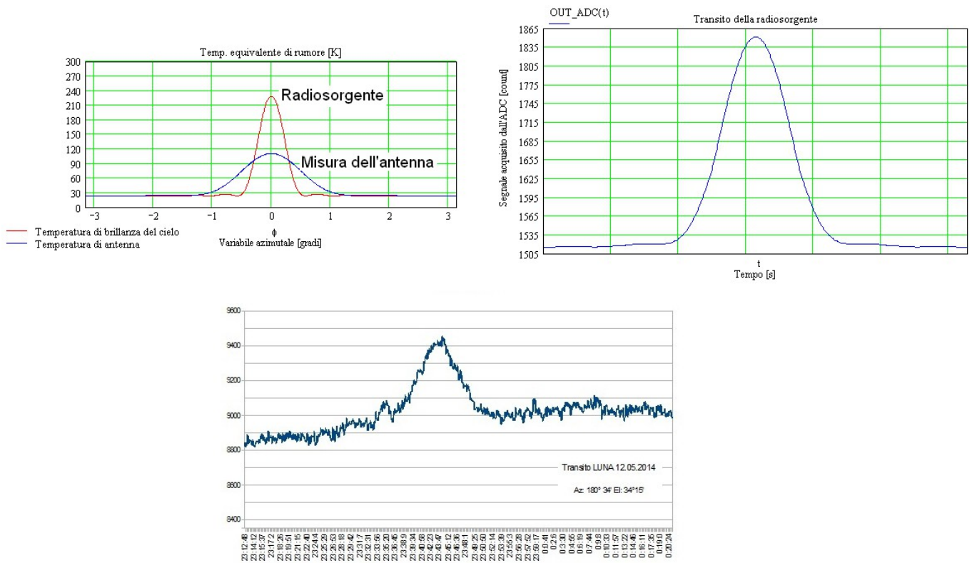
Fig. 10: Le profil théorique de la luminosité de la Lune (graphique en haut à droite) est déterminé par une relation de convolution entre la température de brillance du scénario et la fonction de gain de l'antenne. L'antenne d'un radiotélescope tend à niveler la distribution de la vraie luminosité observée (graphique sur la gauche): l'ampleur de la distorsion instrumentale est due aux caractéristiques de "filtrage spatial" de l'antenne et est lié à la relation entre l'angle de la taille de faisceau de réception et ceux de la source radio apparente. Toute distorsion se produit si le diagramme de réception de l'antenne est très étroit par rapport à l'extension angulaire de la radiosource (le cas de l'antenne très directive). La figure compare l'enregistrement théorique du transit lunaire simulé et un enregistrement expérimental (graphique du bas) effectuée par l'un de nos clients (M. Giancarlo Madai - La Spezia, que nous remercions): à part le niveau de la ligne de base de référence différente, nous pouvons voir que l'amplitude du pic de réception est comparable à celui théorique, estimée à environ 300-350 unités [ADC_count].
