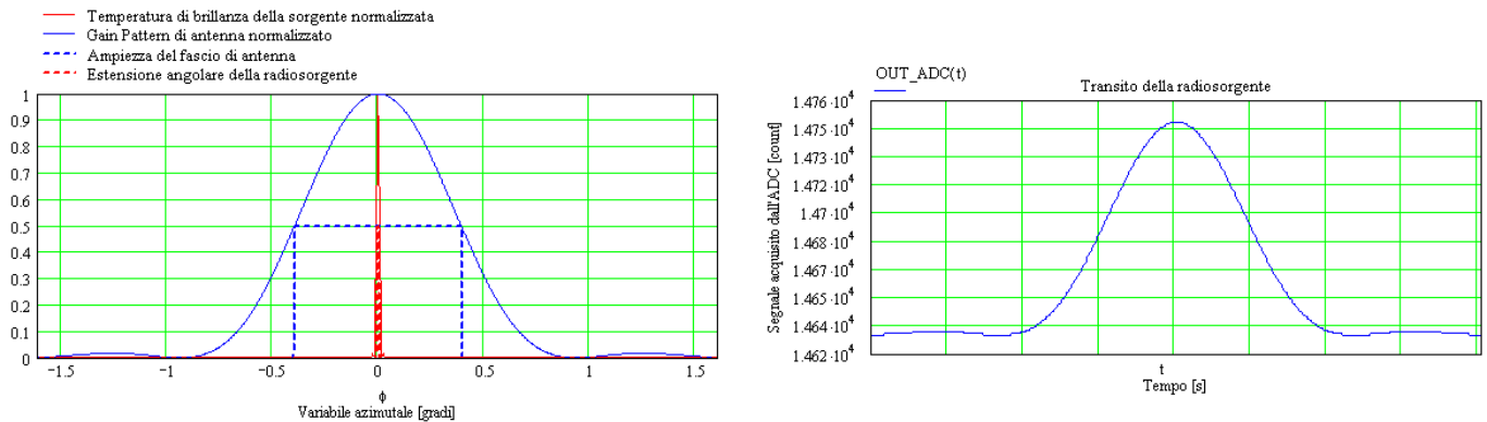
Fig. 12: Simulation théorique du transit de Cassiopee A (3C461) avec une antenne parabolique de réflecteur de 2 mètres de diamètre. On a inséré un amplificateur IF de ligne (12 dB - produit commercial standard utilisé dans les systèmes de réception TV-SAT) reliée à la sortie du LNB pour amplifier la faible variation du signal due à la source radio.
