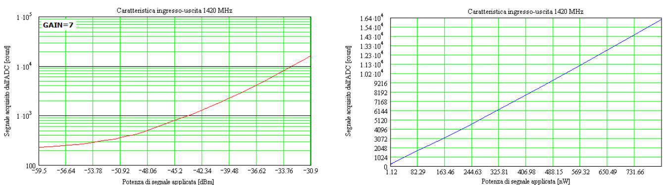
Fig. 7: Caractéristiques d'entrée-sortie du radiomètre obtenues en laboratoire avec un gain post-détection Gain=7 (tension sur les gains égal à 168). L'axe des abscisses indique le niveau du signal RF-FI appliqué, en ordonnée, le niveau de signal acquis par le convertisseur analogique-numérique interne (exprimé en unités relatives [ADC_count]).
