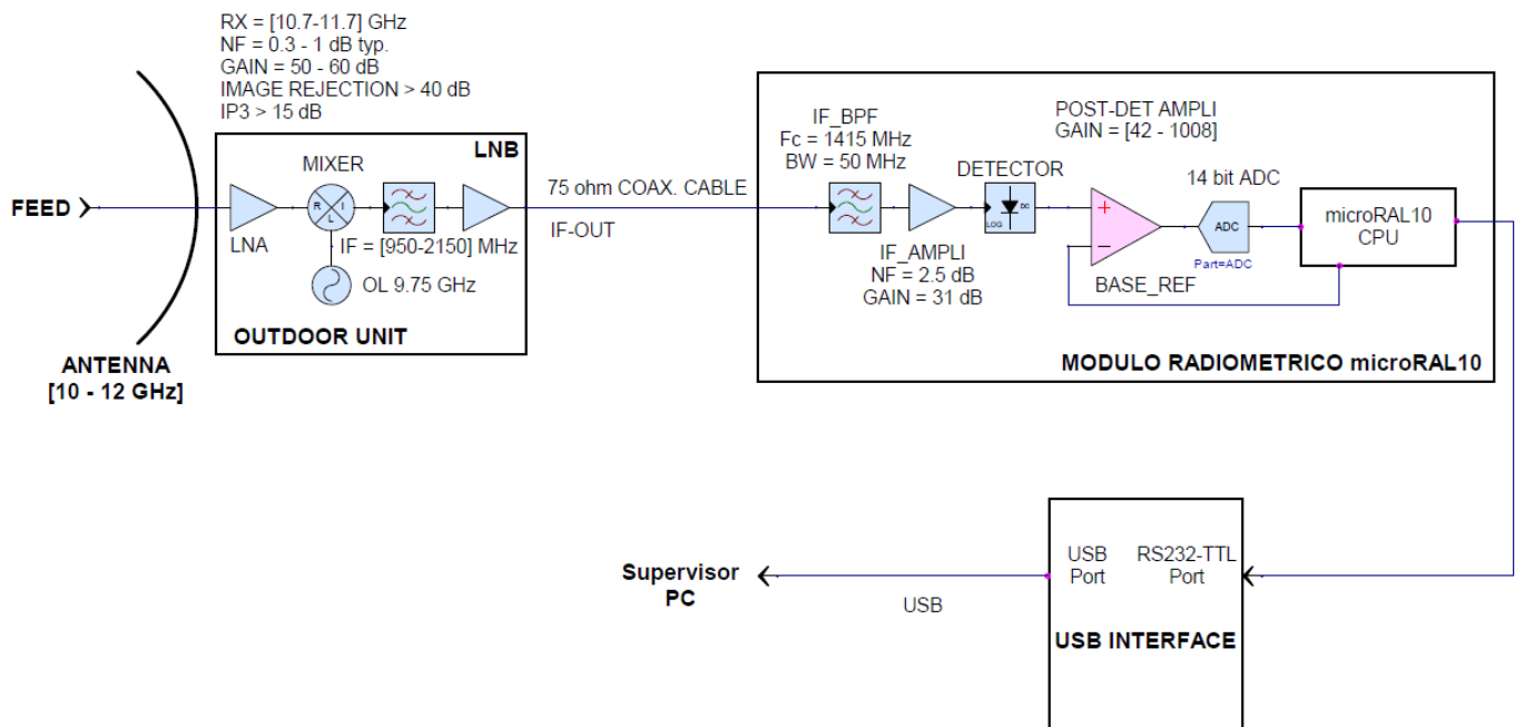
Fig. 4: L'unité extérieure LNB (avec alimentation) est installée au foyer du réflecteur parabolique: un câble coaxial de 75 \Omega TV-SAT relie l'unité extérieure avec le RAL10AP qui communique avec le PC (sur lequel vous avez installé le logiciel DataMicroRAL10 ) à travers une interface USB. Le système utilise un protocole de communication propriétaire. Dans le schéma les circuits audio de sortie d'alimentation et de post-détection ne sont pas représentés. Le récepteur RAL10AP ne comprend pas l'antenne, l'unité extérieure LNB avec alimentation et le câble coaxial de 75 \Omega TV-SAT.
