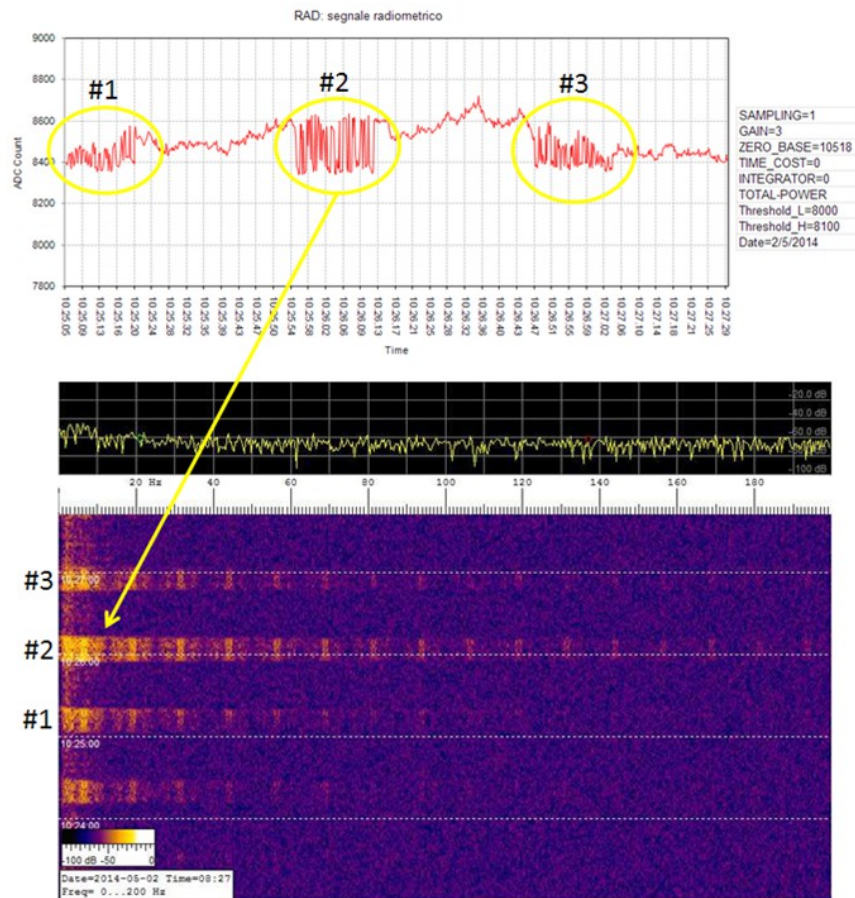
Fig. 9: Les enregistrements réalisés avec RAL10AP . Pour l'expérience, nous avons utilisé l'unité RAL10_LNB extérieur équipé d'une antenne cornet (gain de 20 dB), positionnée sur un trépied photo (en haut à gauche). La sortie du RAL10_LNB a été connectée au récepteur RAL10AP par un câble coaxial. Un PC portable enregistre le signal radiométrique à 11.2 GHz et la réception de données à partir du port USB par le logiciel DataMicroRAL10 (graphique du haut) tandis que simultanément le signal détecteur de son est enregistré ( RAL10AP sortie post-détection audio), il est affiché comme un spectrogramme par le logiciel Spectrum Lab ( http://www.qsl.net/dl4yhf/spectra1.html ).
