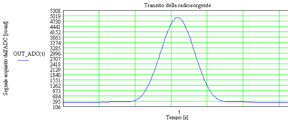
Fig. 11: Simulation du transit du Soleil dans le faisceau de réception du radiotélescope.
